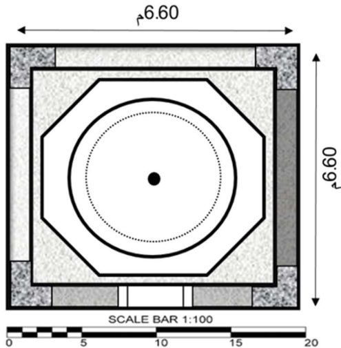
نەخشە ی گۆمەزی بابه شیخ کوری شیخ حسین
