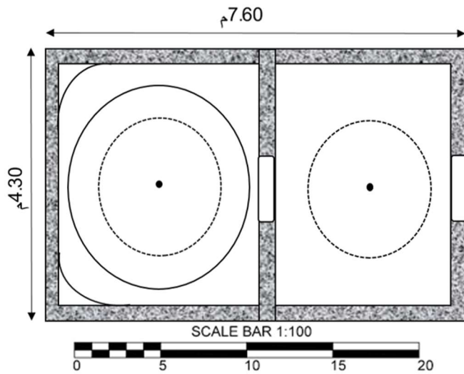
نه‌خشی گلگۆی شیخ شیروان
